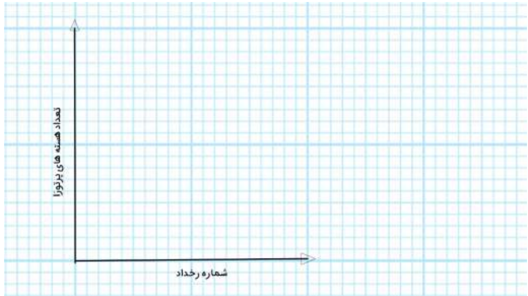
شکل ۳ - نمودار تعداد هسته های پرتو زا در هر مرحله پرتاب تاس
