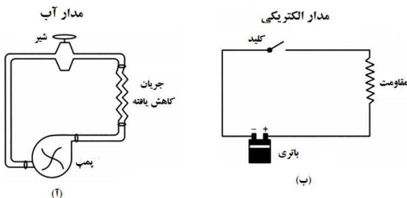
شکل 1. مقایسه یک مدار آب (آ) و یک مدار الکتریکی (ب).
