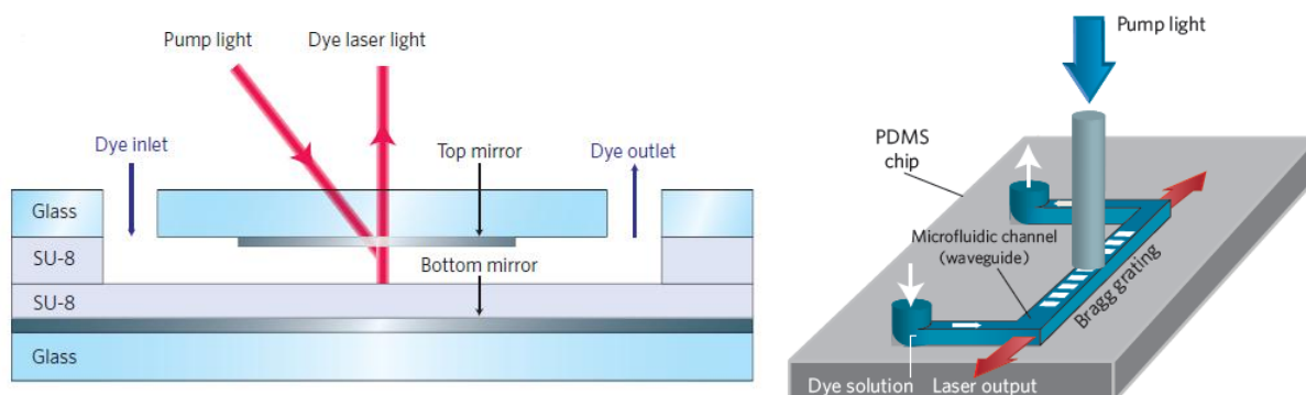
شکل ۱۰: طرح واره‌ای از لیزر اپتوفلودیک (الف) لیزر کاواک عمودی [۸] لیزر بازخورد توزیع شده با دمش عمودی [۹].
