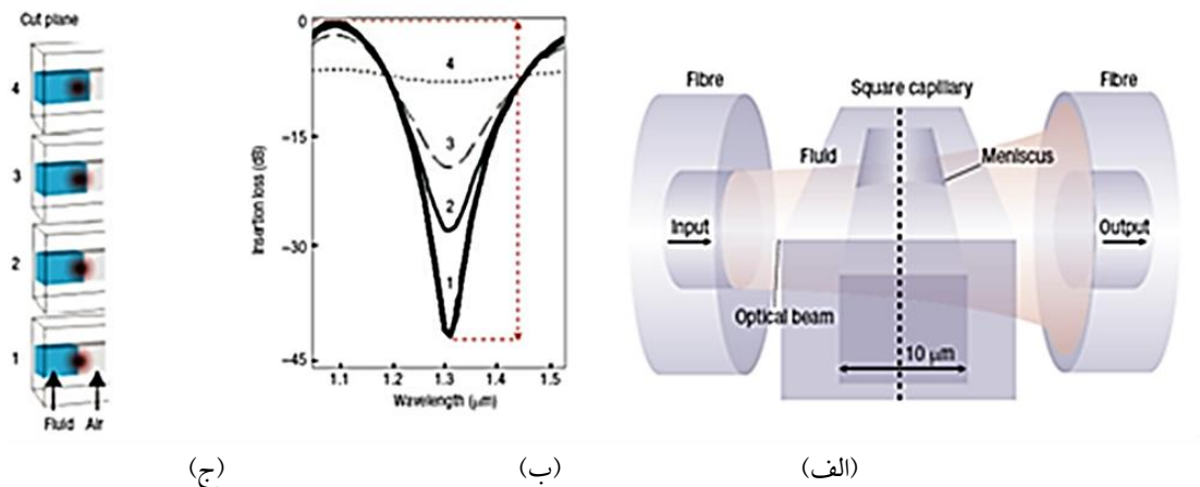
شکل ۸: (الف) طرح واره-ای از تداخل سنج تک باریکه-ای (ب) تغییرات طیف تراگیسل افزاره (ج) چگونگی تنظیم پذیری تداخل سنج، با حرکت مرز بین آب-هوا نسبت به مرکز باریکه [۱۵].
